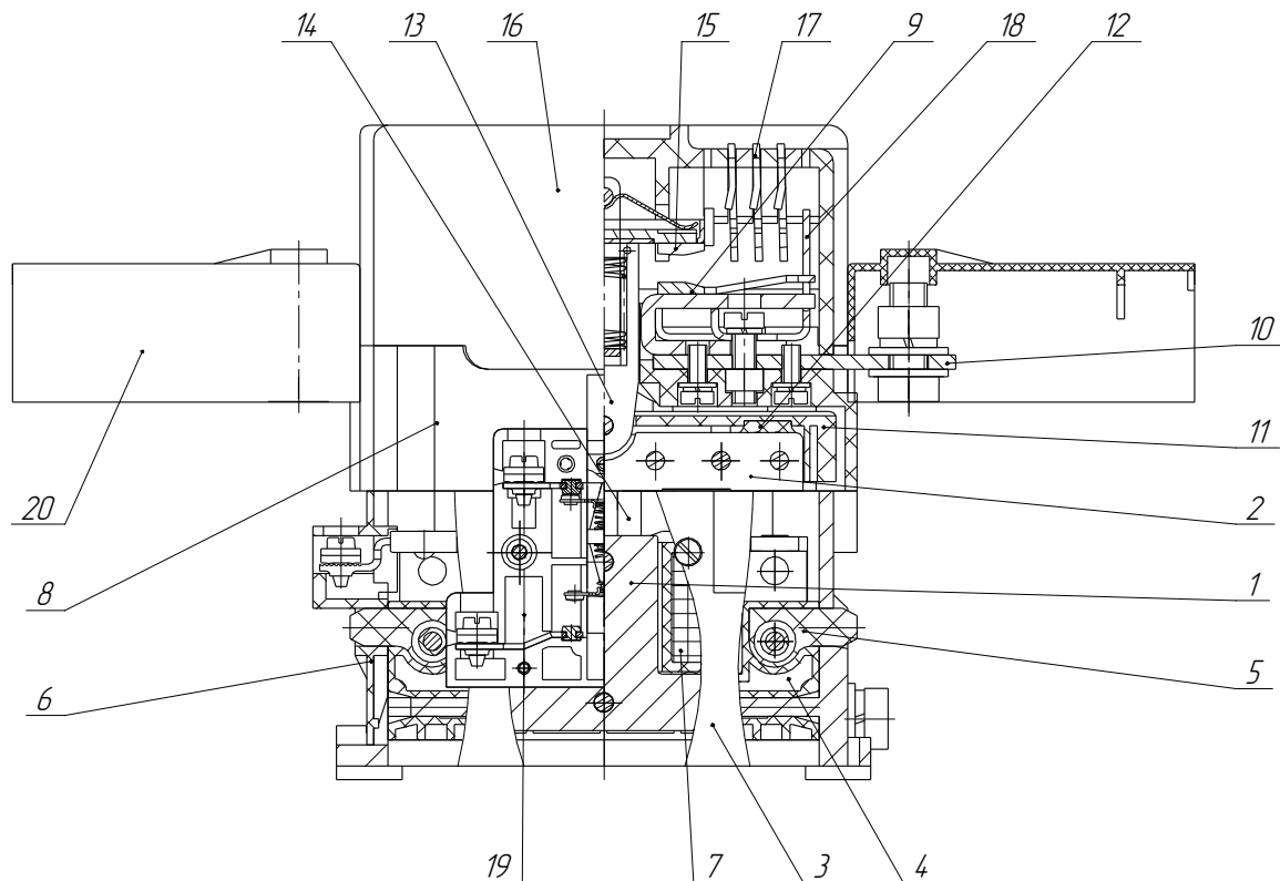
Рисунок 1 - Контактор неперевсивный ПМЛ-5101; ПМЛ-5161; ПМЛ-5101Д; ПМЛ-5161Д
