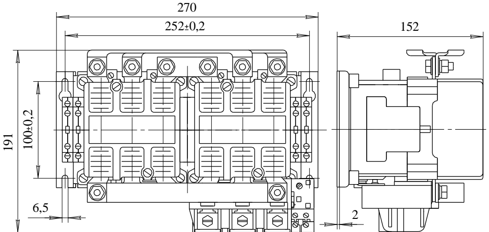
Рисунок Б.3 - Контакторы реверсивные ПМЛ-5501Д, ПМЛ-5501
