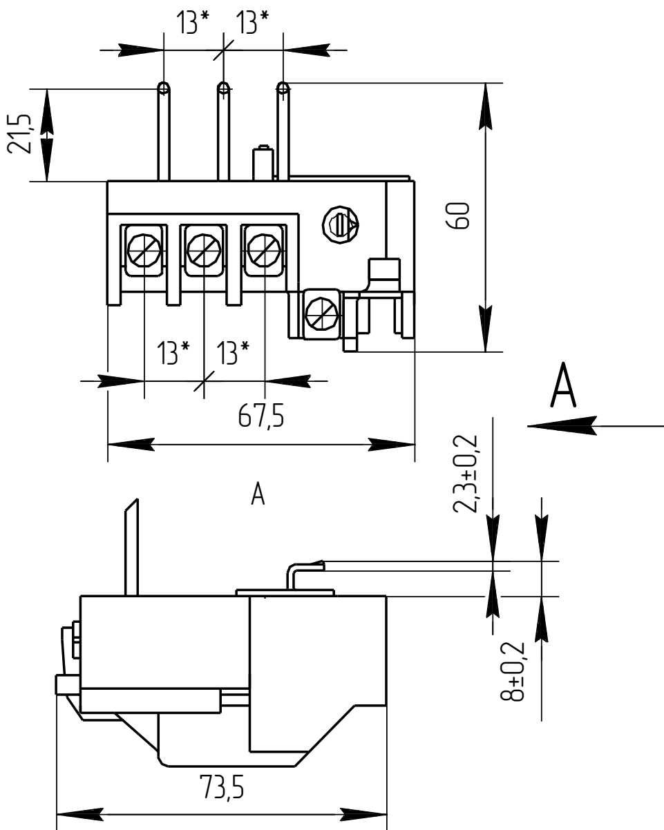
Рисунок Б.3 — Реле типов РТТ-131, РТТ-13. Масса реле не более 0,155 кг.
