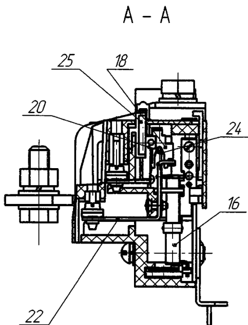
Рисунок 2 - Реле РТТ5-180
