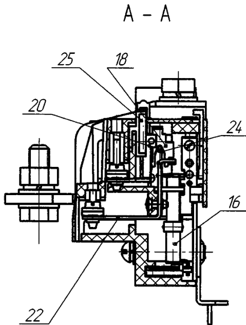
Рисунок 2 - Реле РТТ5-180
