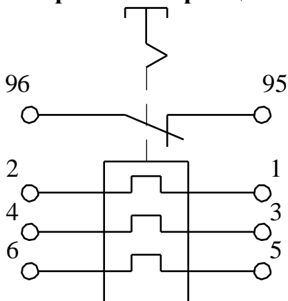
Рисунок В 1 - Реле с размыкающим контактом
