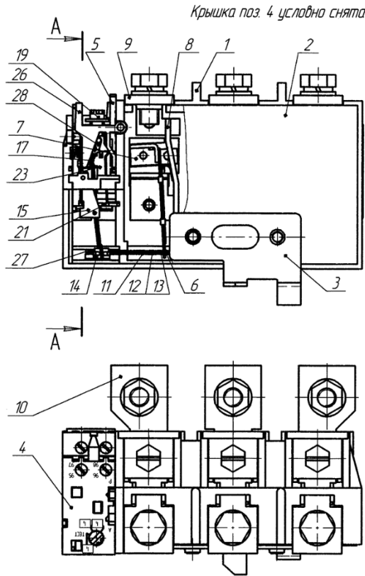
Рисунок 1- Реле РТТ5-180
